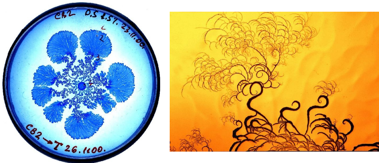
FIGURA 6: Formaciones fractales de colonias bacterianas.
