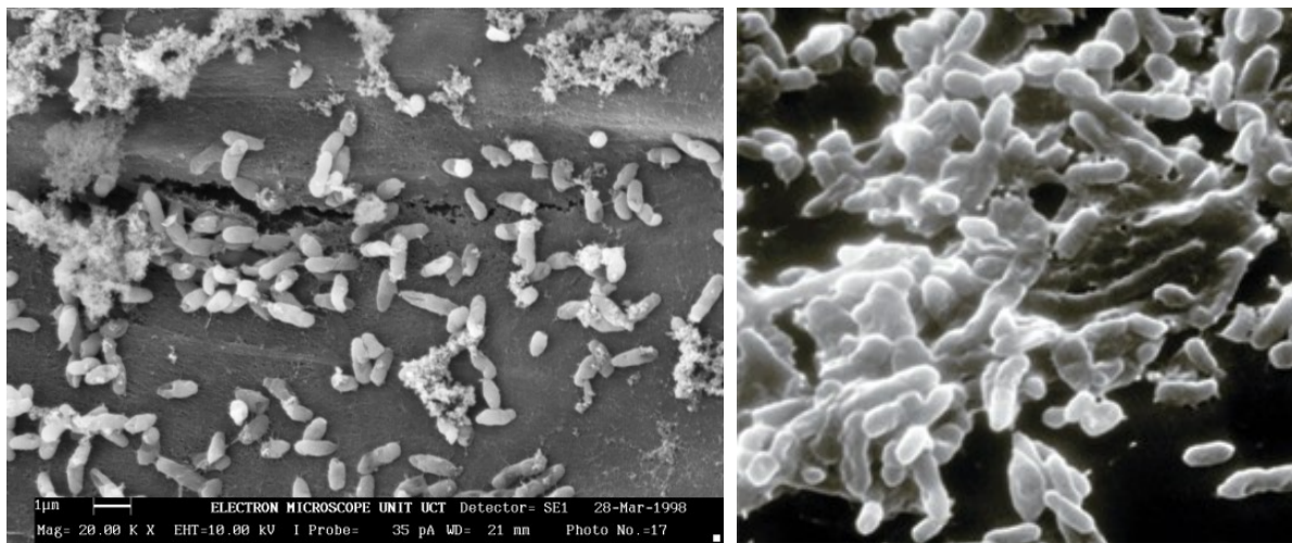
FIGURA 5: Fotos de bacterias a través del microscopio electrónico.
