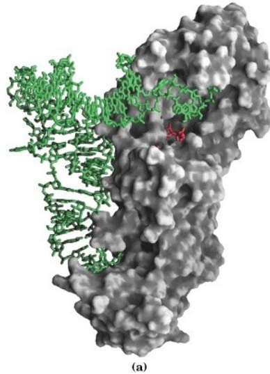
(a) FIGURA 4: Representación tridimensional de la enzima aminoacil-tRNA sintetasa interpretando una secuencia de ADN.
